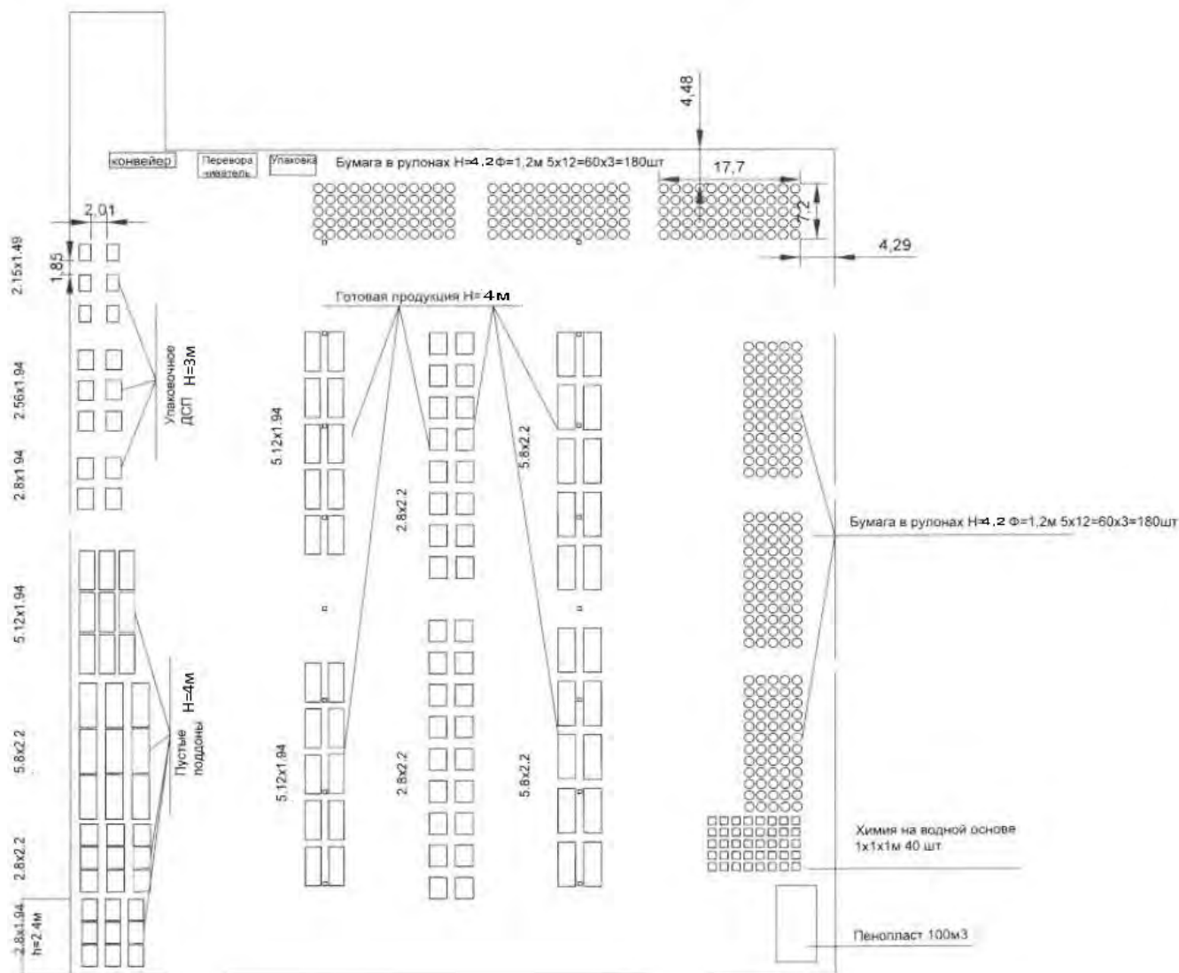
Рисунок 1.2.1 – Схема складирования
