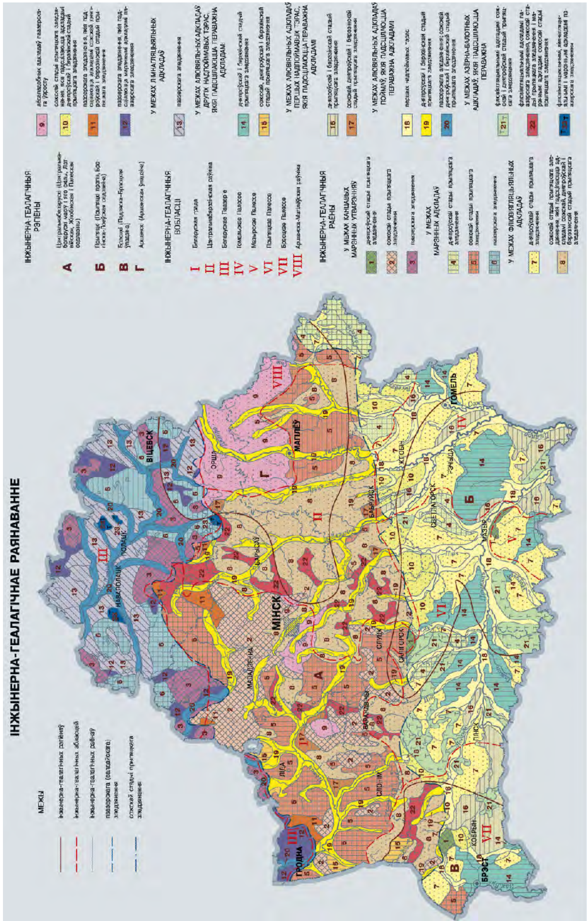
Рисунок 4.1.4.5 – Карта инженерно-геологического районирования территории Беларуси (заимствована из Национального Атласа Беларуси) [26]
