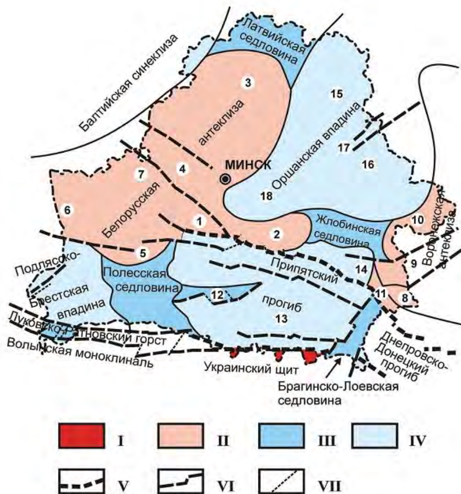
Рисунок 4.1.4.2 – Карта тектонического районирования территории Беларуси [26]
