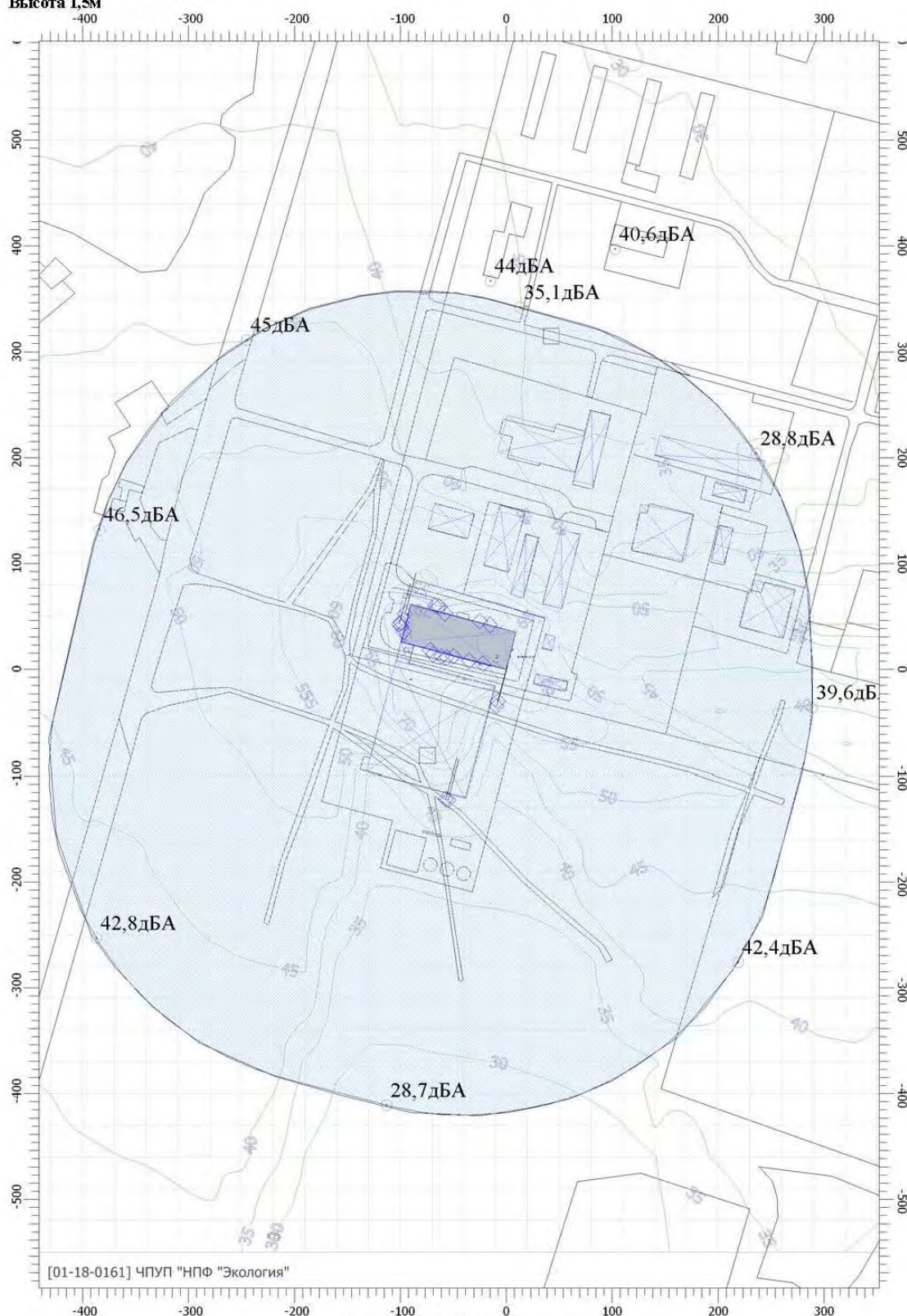
Рисунок 6.2.1 – Карта расчетных эквивалентных уровней звука в расчетных точках на границе СЗЗ и в жилой зоне
